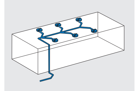
↑ Geberit Pluvia sifonik çatı drenaj sistemi
