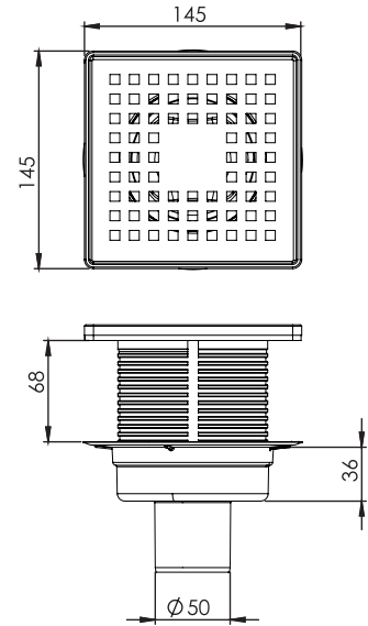
15*15 Dikey Sifon
