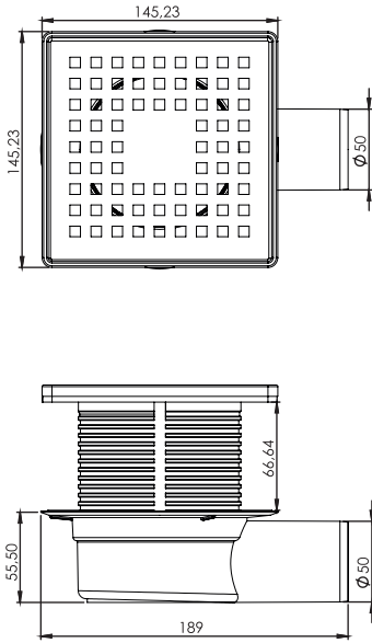
15*15 Yatay Sifon
